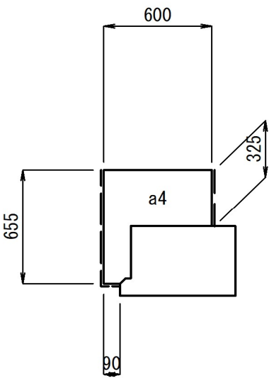
A2側桁端部
