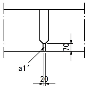
支点断面変化部
