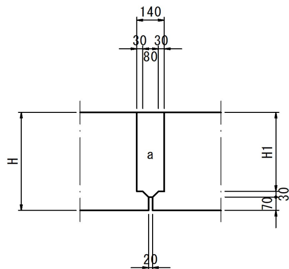
中間横桁部
